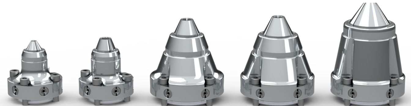
W15 bis zu Ø16 mm W20 bis zu Ø20 mm W25 bis zu Ø25 mm B32 bis zu Ø28 mm B32/45 bis zu Ø40 mm
